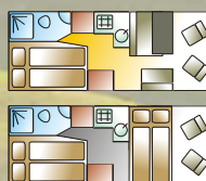
i 780 Fiat Ducato 33L 3,30to - 6,93m 96kW(130PS) 2,3 Multijet
